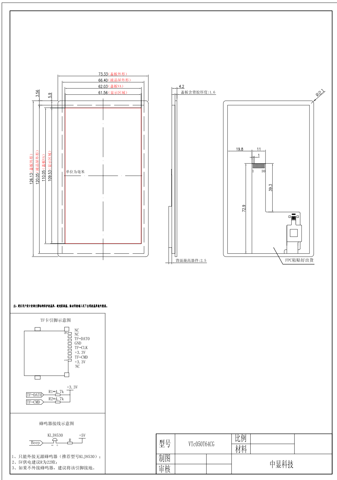
图 3 VTc050T64CG 尺寸图
